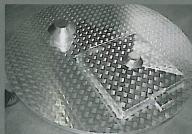
Ø2000 mm alu-dæksel med 800 x 800 mm mandehul
